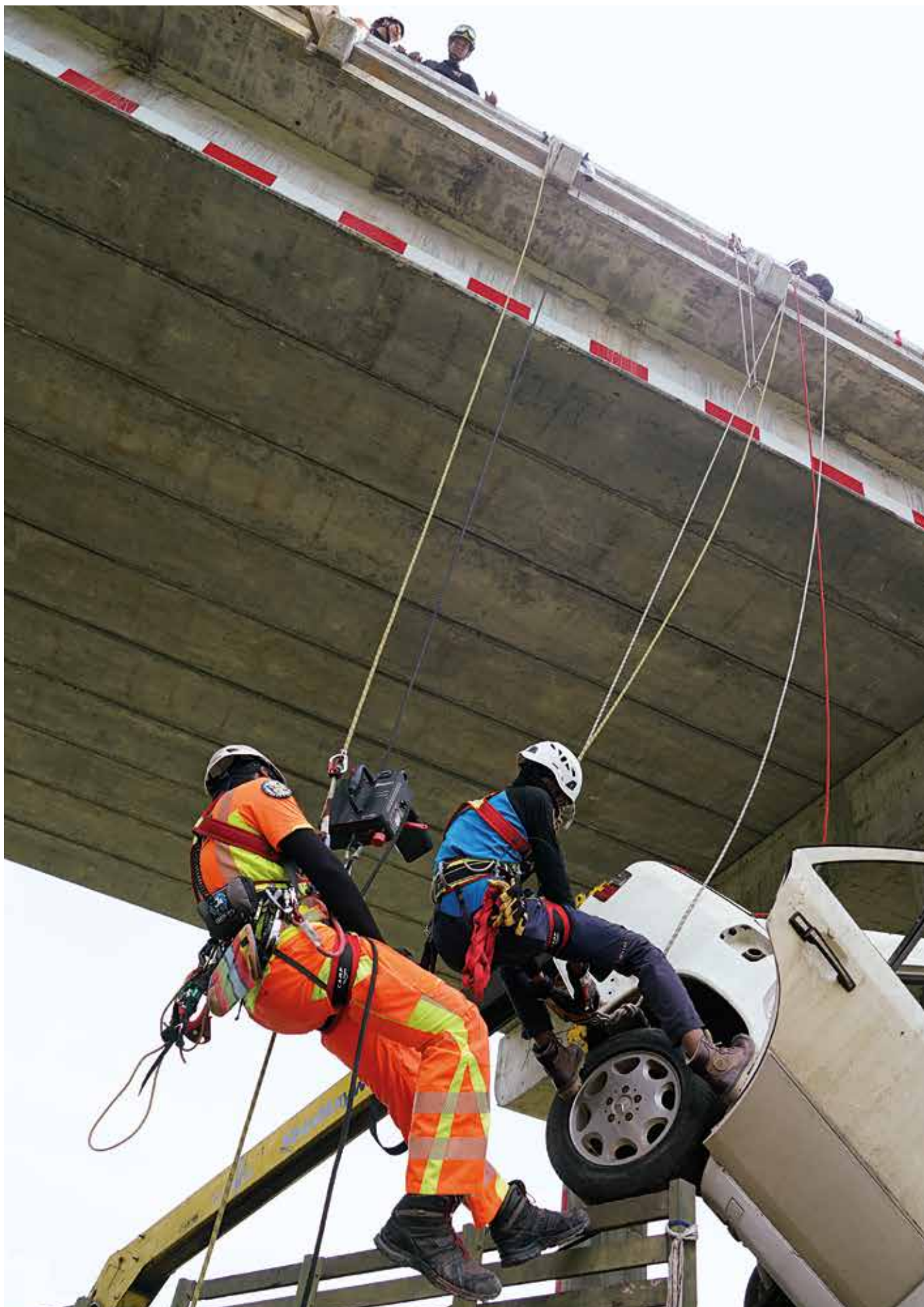
A "FROG Team" member demonstrating a rope rescue. Un miembro del "Frog Team" haciendo una demostración de rescate por cuerdas. Surat Thani, Bangkok, Thailand (courtesy of Outdoor Solution Co. Ltd., ph. Pi-Ti Praomatooros).
