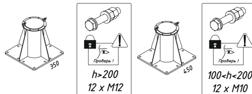
Рисунок 3 - Монтаж базы опорной (горизонтальной) vpro E012-6-F-***
