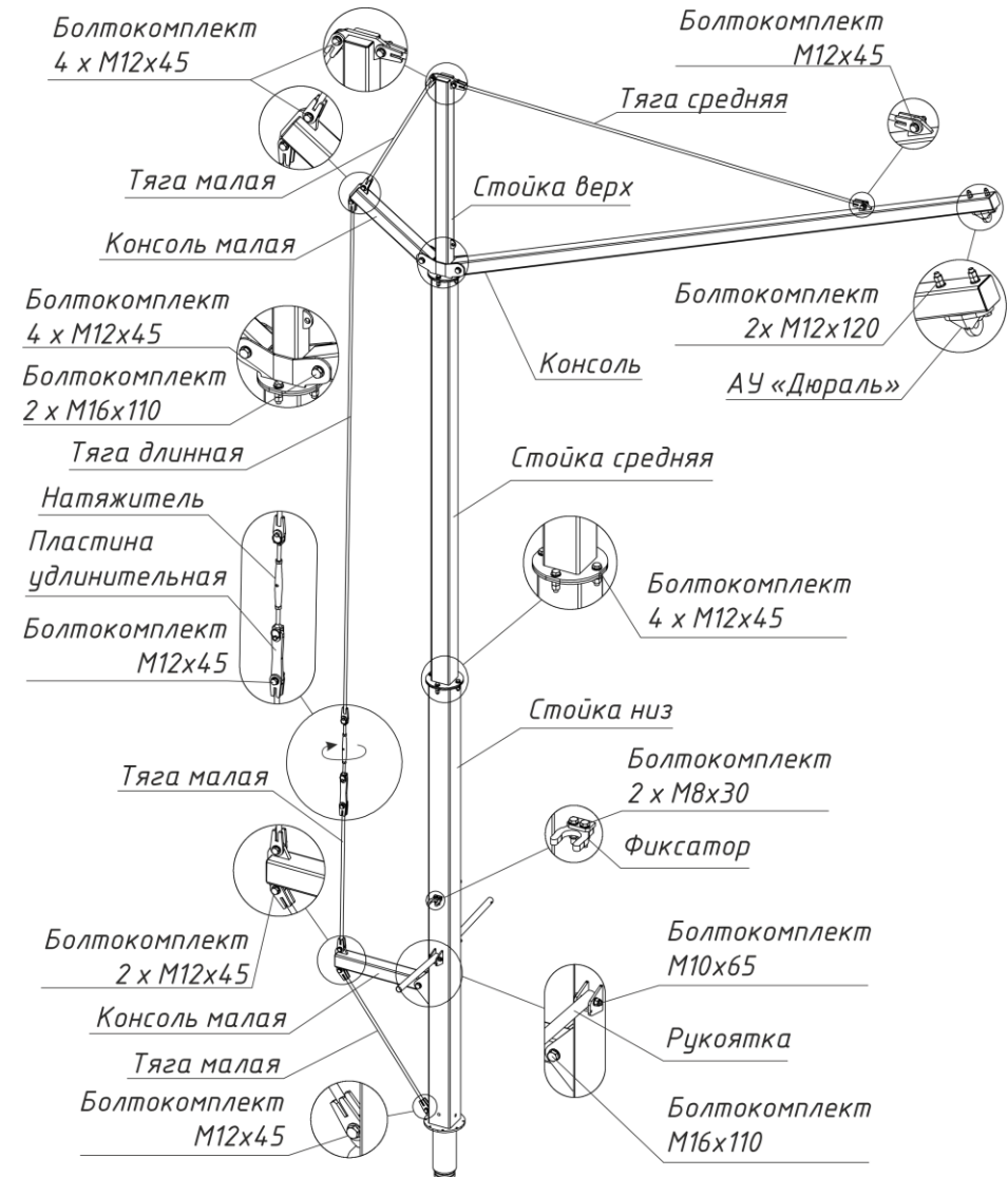
Рисунок 4 – Монтаж стойки vpro E012-6-* СОБ Вентпро Е12-6-*
