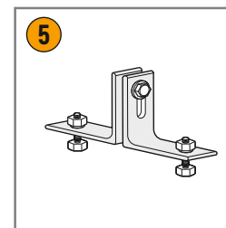
RHL44 СТРУКТУРНЫЙ АНКЕР
