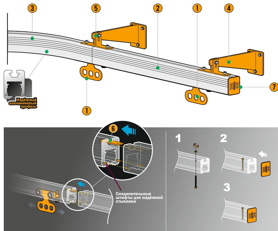
Рис. 1 Горизонтальная жесткая анкерная линия AVRORA.
