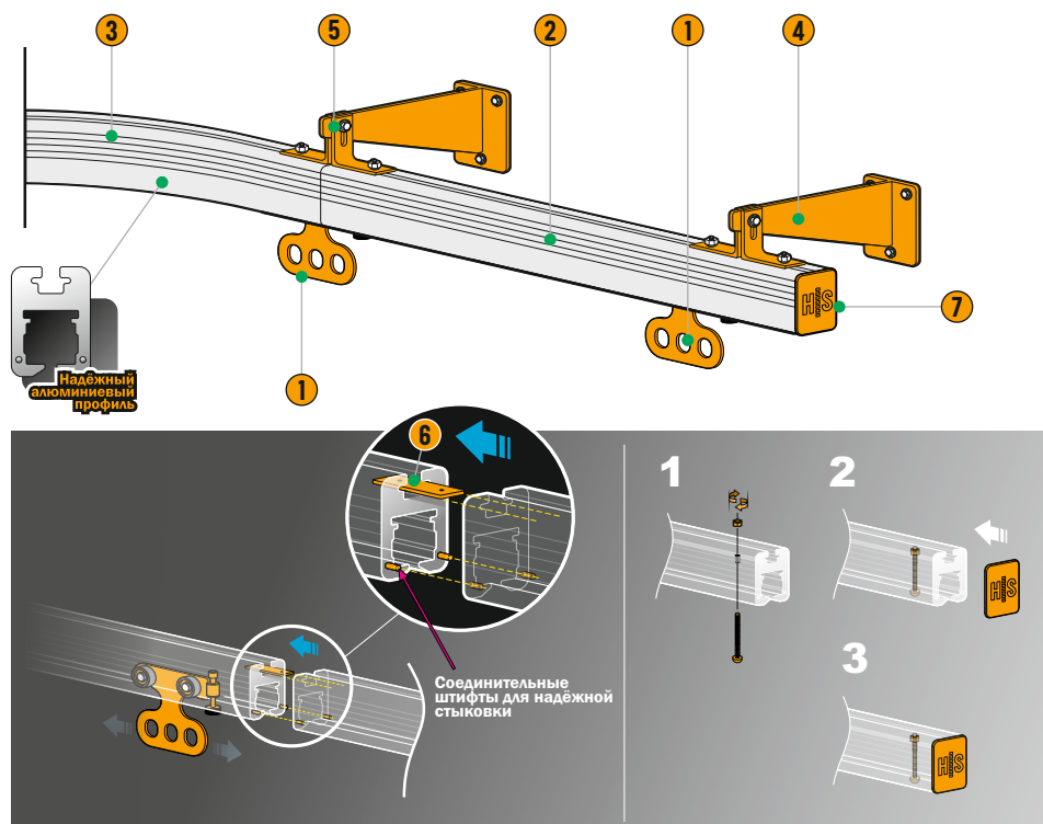
Рис. 1 Горизонтальная жесткая анкерная линия AVRORA.
