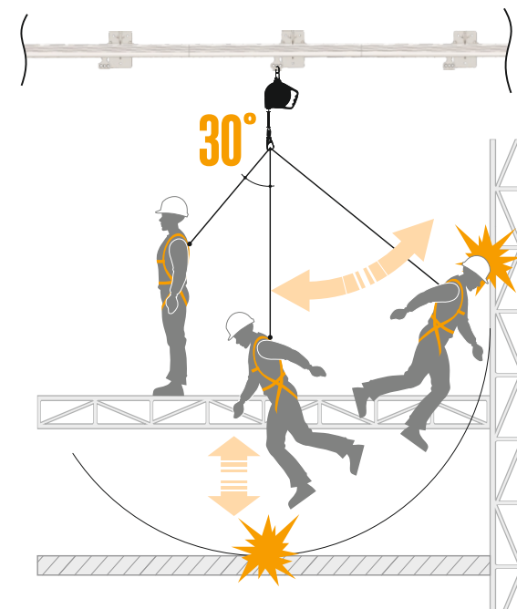
Рис. 5 Падение работника, сопровождающееся маятниковым движением.
